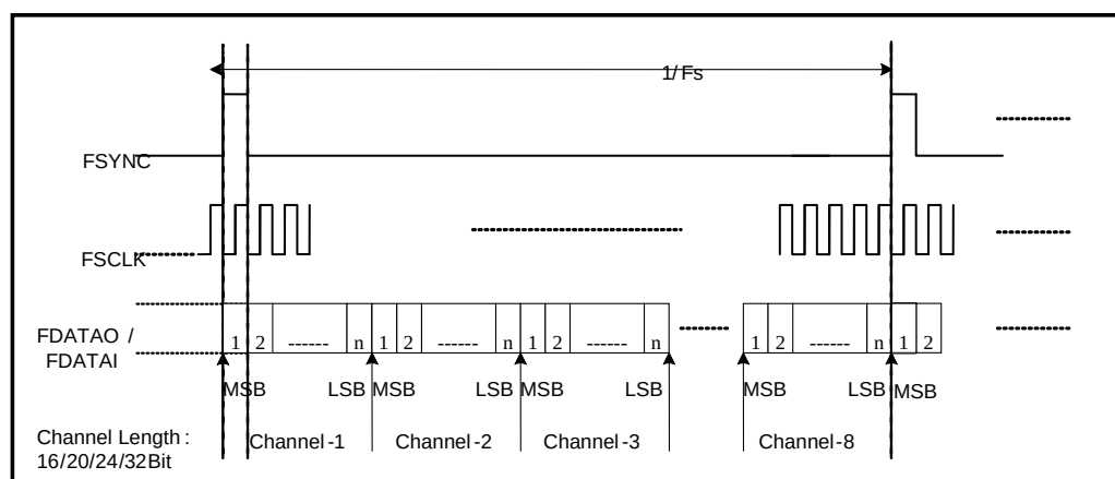
Fig. 7.6.2 TDM Mode 2
